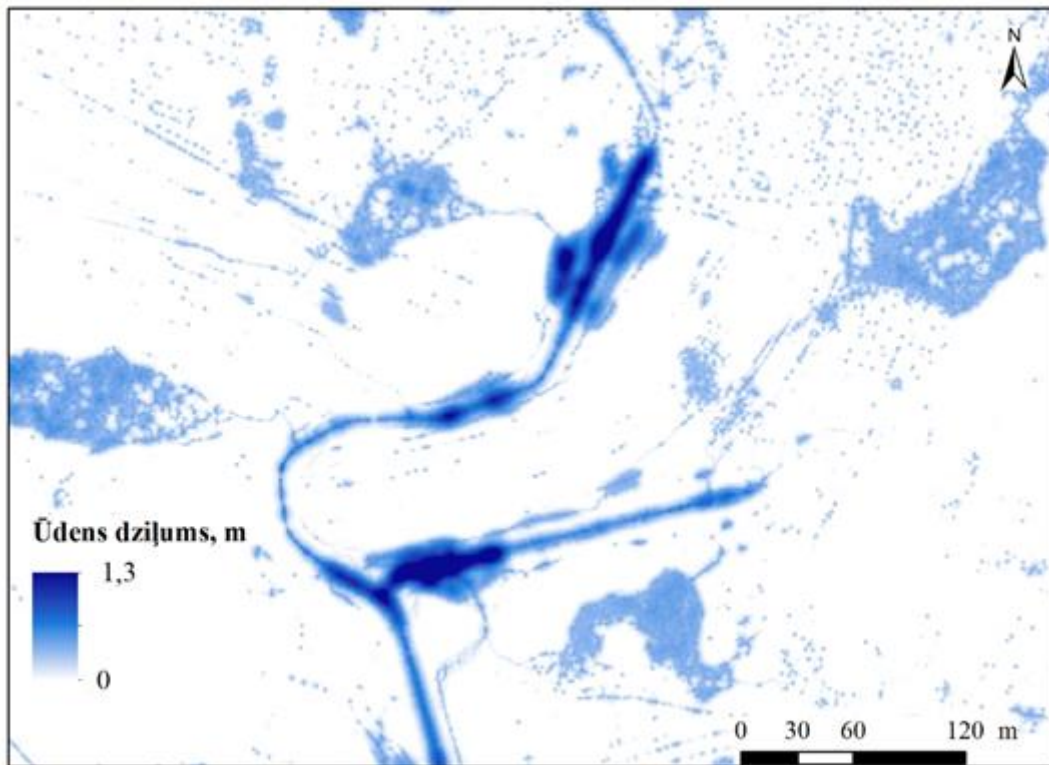
3.3. attēls. Modelētā ( 15 \text{ mm h}^{-1} , 10 h) nokrišņu ūdens akumulācija Bērze teritorijā.
