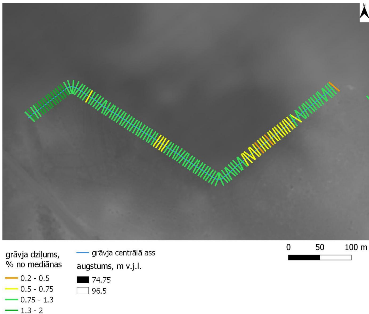
3.4. attēls. Grāvju šķēršprofilu analīzes vizuāls piemērs.
