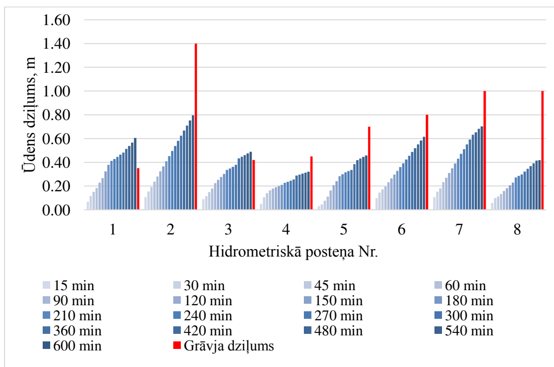
3.2. attēls. Ūdens dziļums hidrometriskajos posteņos Bērzes paraugteritorijā.
