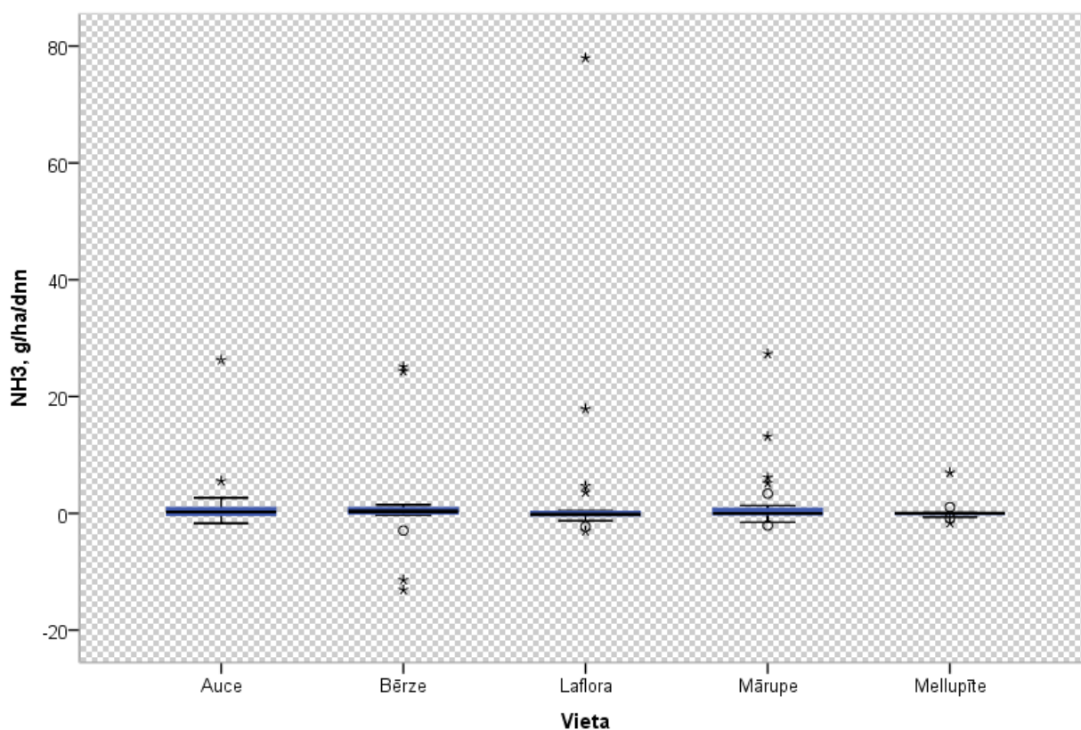
23.att. \text{NH}_3 emisiju novērojumi pētījumu objektos 2020. gadā.
