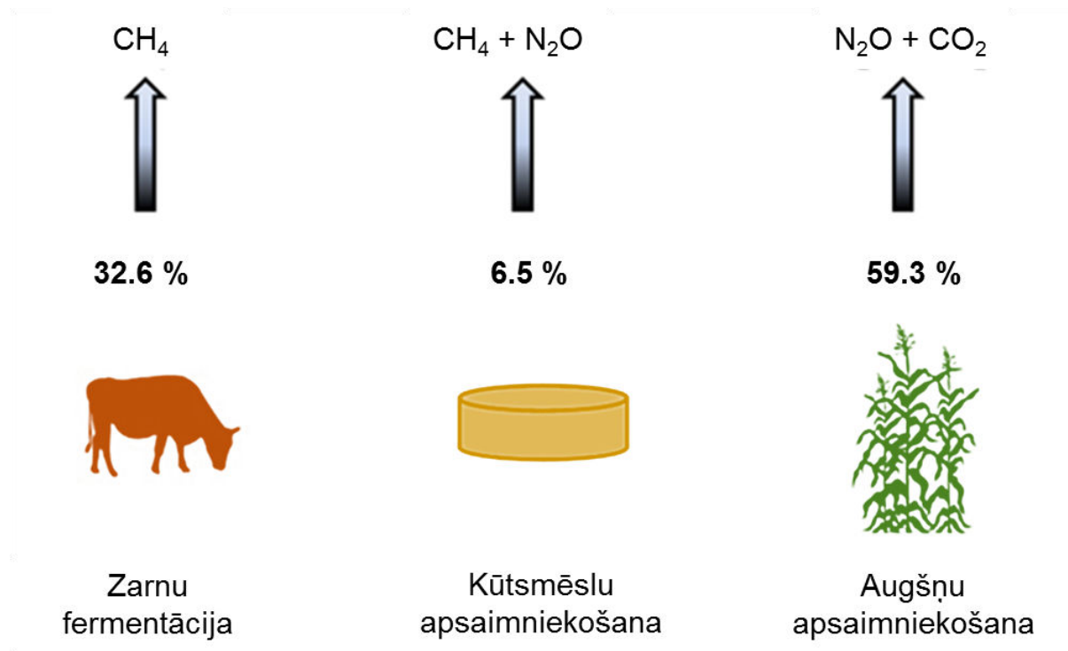
4. att. Galvenie SEG emisiju avoti lauksaimniecībā 2018. gadā (NIR, 2020).
