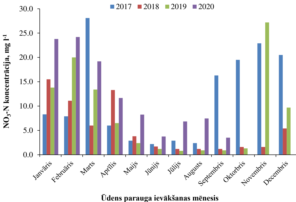
6. attēls. Nitrātu – slāpekļa koncentrācijas Vecauces sateces baseina (VecauceSC) monitoringa postenī 2017., 2018., 2019., 2020. gadā ievāktajos ūdens paraugos.
