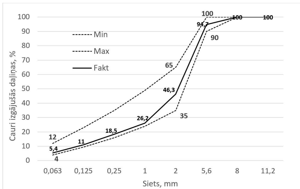
25. att. DSK 5 granulometriskā sastāva atbilstība reglamentētajām robežām
