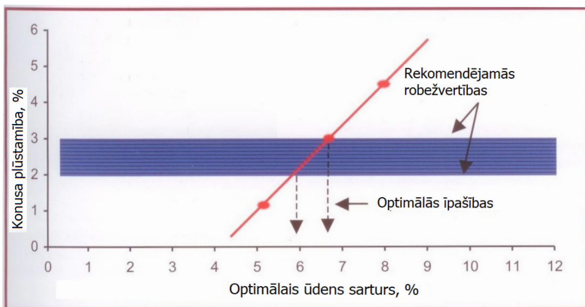
8. att. Optimālā ūdens saturs noteikšana ar konusa nosēduma testu (USIRF)
