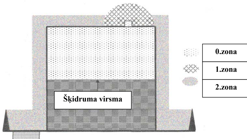
Attēls 3.4. Piemērs, kā klasificē zonas pie tvertnēm, kuras satur uzliesmojošus šķidrumus.
