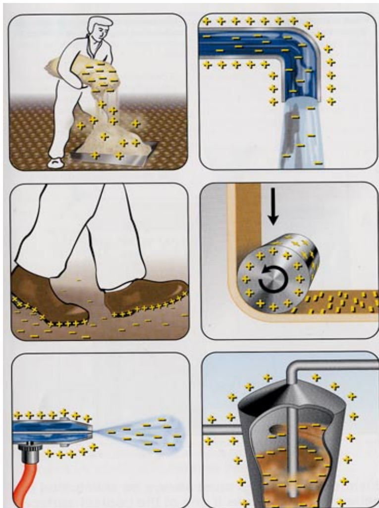
Attēls 3.6. Dažādu sadalīšanās procesu piemēri, kas var radīt elektrostātiskos lādiņus. 5
