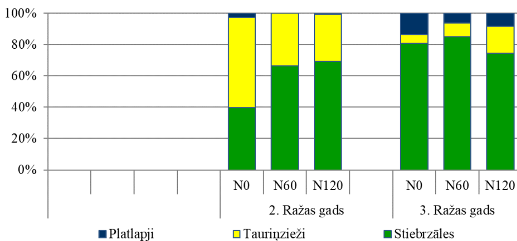
44. att. Stiebrzāļu – tauriņziežu kombinētās izmantošanas zemeņu pirmā plāvuma botāniskais sastāvs divos izmantošanas gados (%), Vecauce
