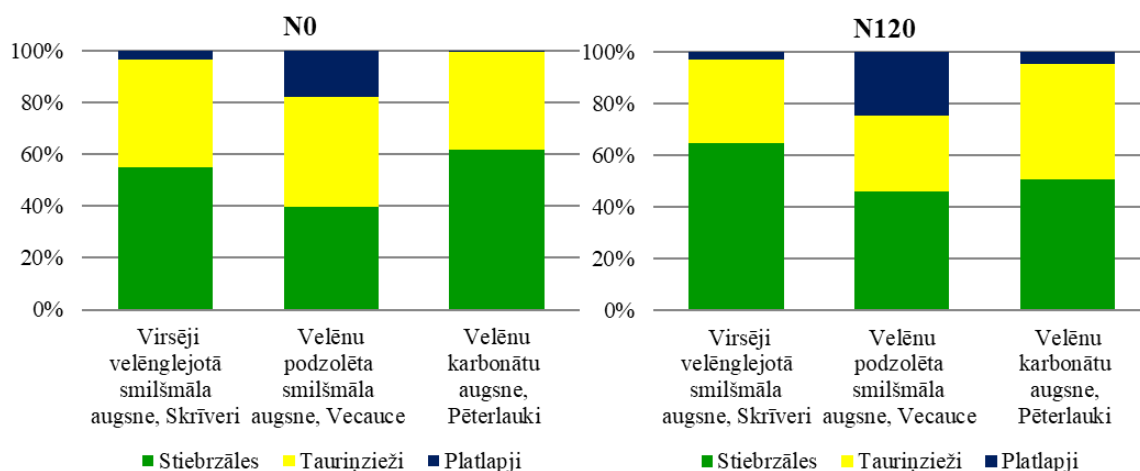
16. att. Stiebrzāļu – tauriņziežu ganību zelmeņu pirmā plāvuma botāniskais sastāvs (%)
