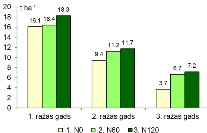
41. att. Kombinētās izmantošanas zelnepu sausnas raža trijos ražas gados (Vecauce), t ha -1
