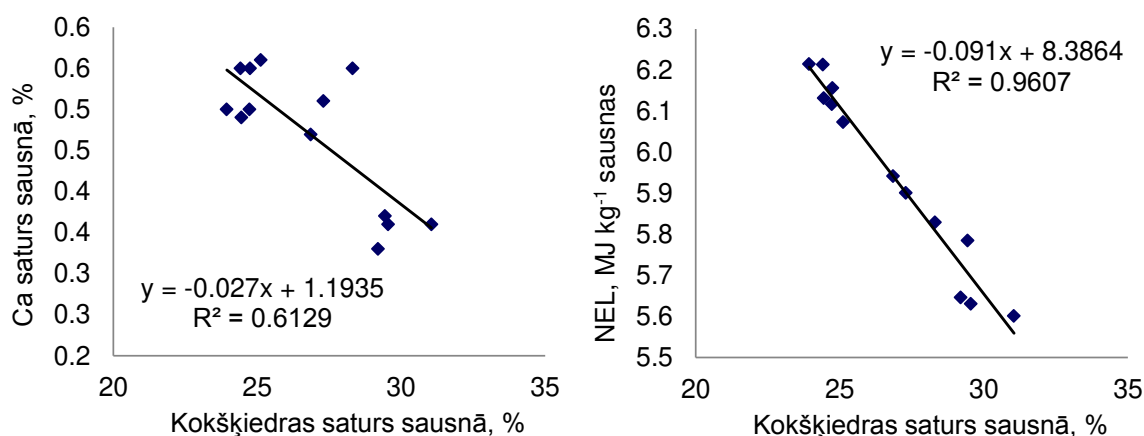
51. att. Korelatīvā sakarība starp NEL, Ca saturu saunā un kokšķiedras saturu saunā kombinētās izmantošanas zelmeņos Vecaucē
