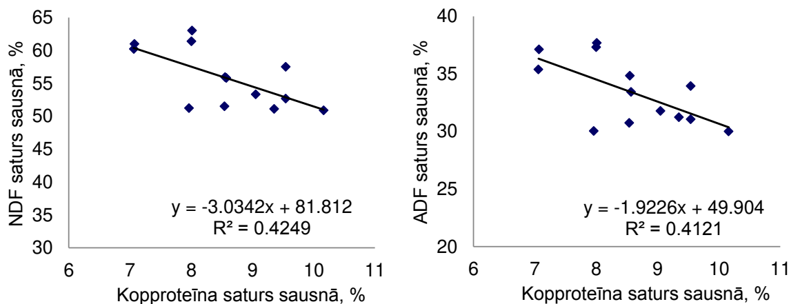
50. att. Korelatīvā sakarība starp kopproteīna saturu saunā un kokšķiedras frakcijām kombinētās izmantošanas zelmeņos Vecaucē
