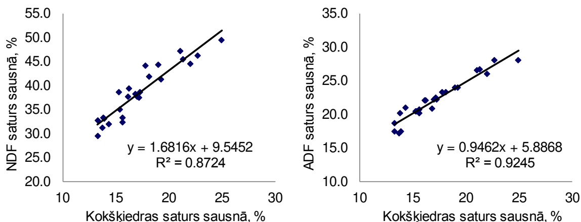
23. att. Korelatīvā sakarība starp kokšķiedras saturu un kokšķiedras frakcijām NDF un ADF ganību zelmeņos Pēterlaukos
