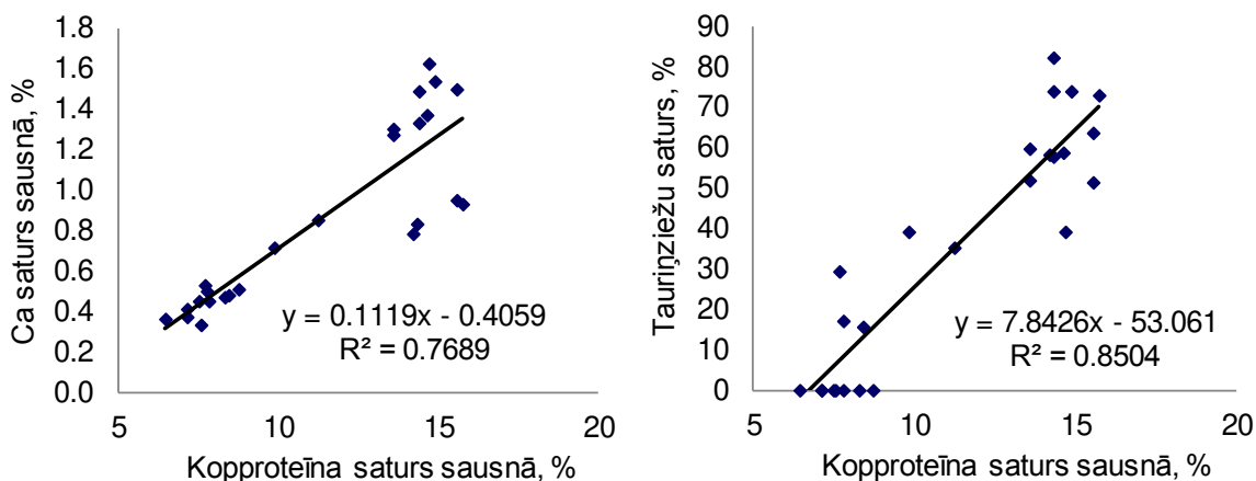
35. att. Korelatīvā sakarība starp tauriņziežu saturu, Ca saturu saussnā un kopproteīna saturu pļaušanas zelmeņos Vecaucē
