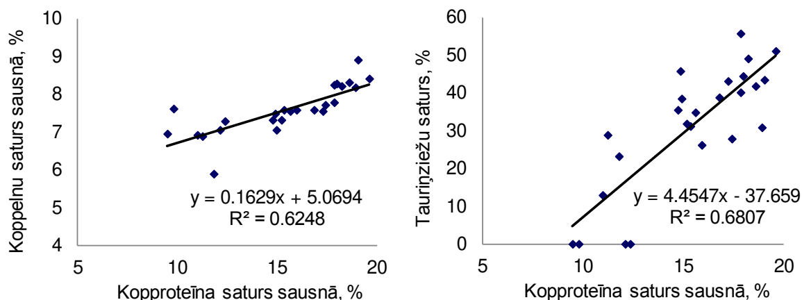
18. att. Korelatīvā sakarība starp tauriņziežu saturu, koppelnu saturu sausnā un kopproteīna saturu ganību zelmeņos Skrīveros
