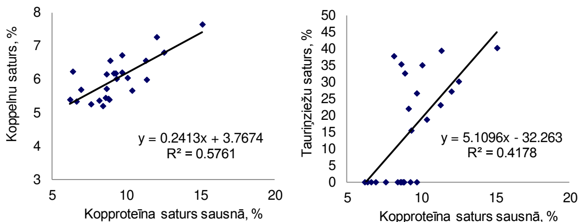
33. att. Korelatīvā sakarība starp tauriņziežu saturu, koppeļu saturu saussnā un kopproteīna saturu pļaušanas zelmeņos Skrīveros
