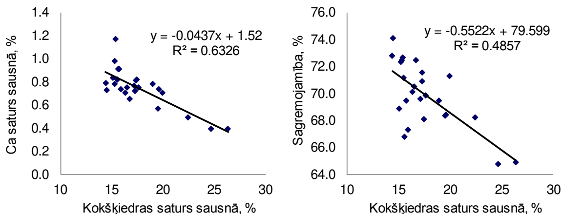
21. att. Korelatīvā sakarība starp Ca saturu, sausas sagremojamību un kokšķiedras saturu sausnā ganību blokā Vecaucē
