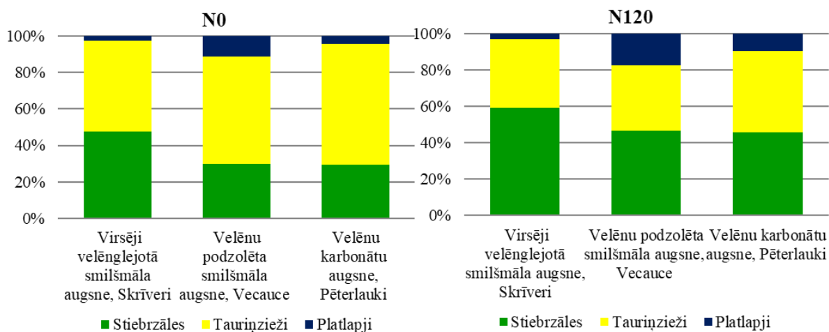
17. att. Stiebrzāļu – tauriņziežu ganību zelmeņu otrā plāvuma botāniskais sastāvs (%)
