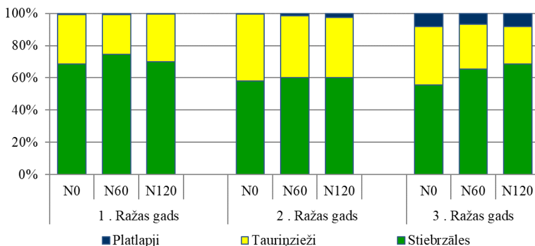
43 att. Stiebrzāļu – tauriņziežu kombinētās izmantošanas zelmeņu pirmā plāvuma botāniskais sastāvs trijos izmantošanas gados (%), Skrīveri
