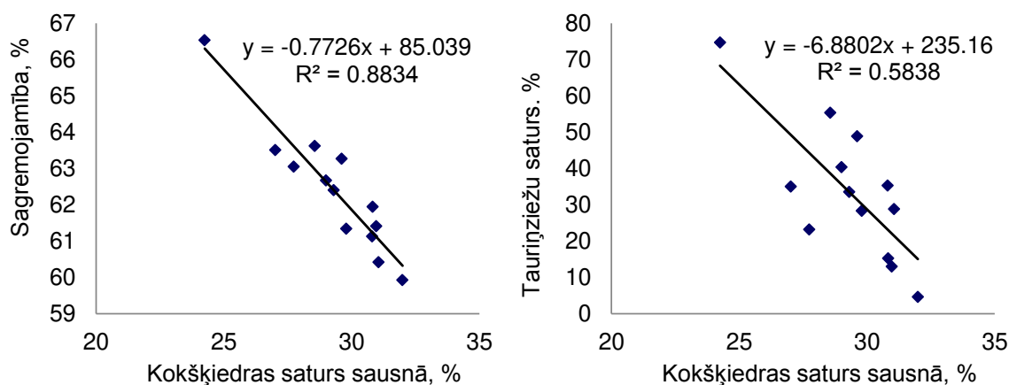
53. att. Korelatīvā sakarība starp tauriņziežu saturu, sausas sagremojamību un kokšķiedras saturu sausnā kombinētās izmantošanas zelmeņos Pēterlaukos
