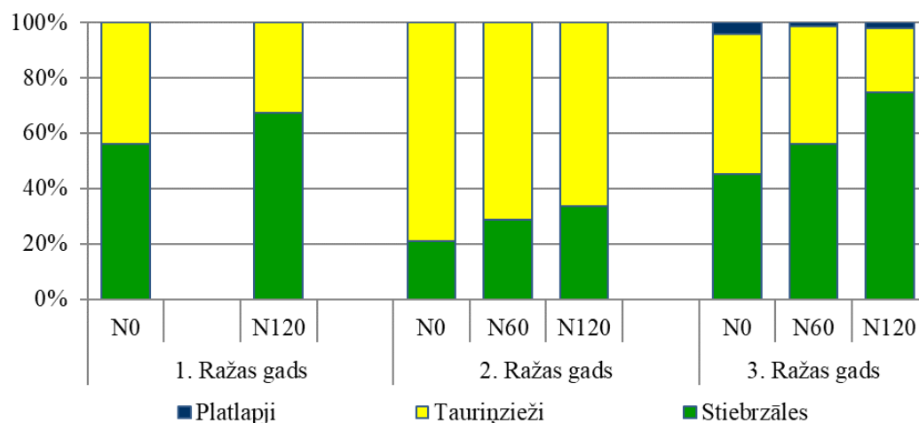
45. att. Stiebrzāļu – tauriņziežu kombinētās izmantošanas zelmeņu pirmā plāvuma botāniskais sastāvs trijos izmantošanas gados (%), Pēterlauki
