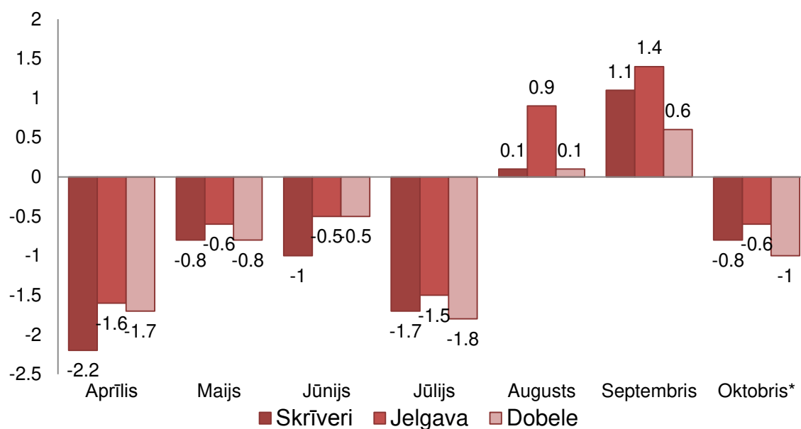
7. att. Vidējās gaisa temperatūras novirze no mēneša normas, °C
