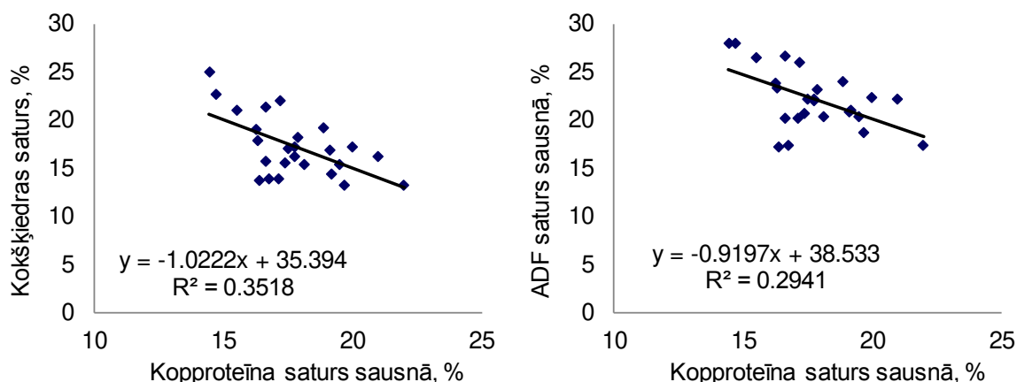
22. att. Korelatīvā sakarība starp kopējās kokšķiedras saturu, ADF saturu saussnā un kopproteīna saturu un ganību zelmeņos Pēterlaukos
