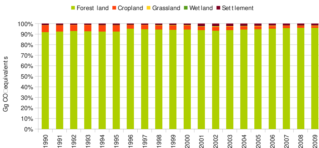
Att. 30 Neto emisiju absolūto vērtību summa 1990.-2009. gadā (LVĢMC 2011).
