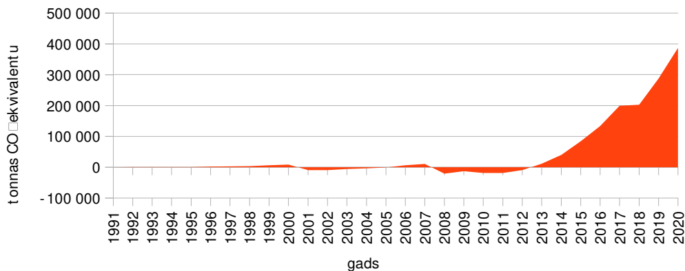
Att. 33 Atšķirības CO 2 piesaistē scenārijā “ar pasākumiem” un “ar papildus pasākumiem”
