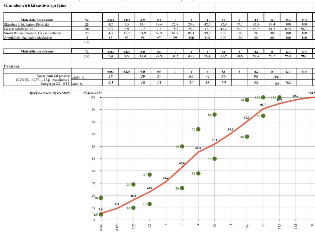
4-7 tabula. Granulometriskais sastāvs (LVS EN 933-1) – reciklētais sastāvs 0/16 ar frēzētu asfaltu, šķembu maisījumu un smilti, aprēķins
