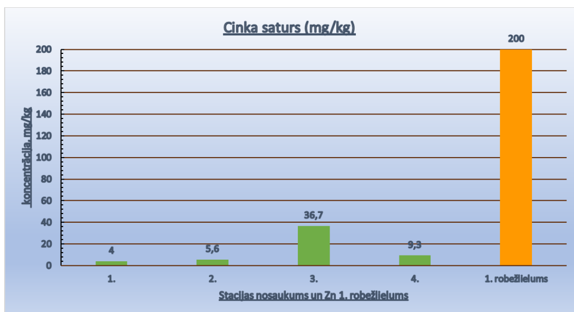
Grafiks Nr.2 Cinka saturs
