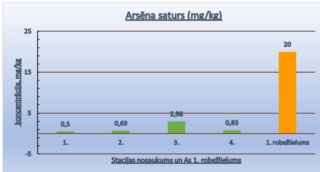
Grafiks Nr.8 Arsēna saturs
