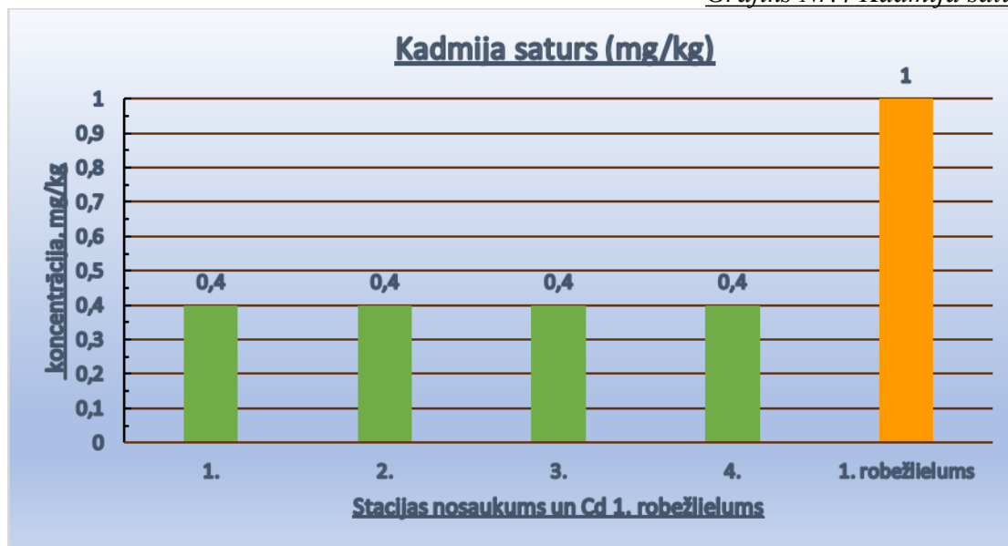
Grafiks Nr.4 Kadmija saturs
