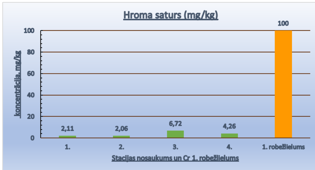
Grafiks Nr. 6 Hroma saturs
