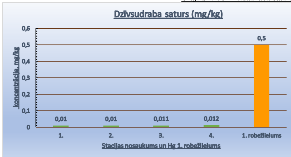
Grafiks Nr. 3 Dzīvsudraba saturs
