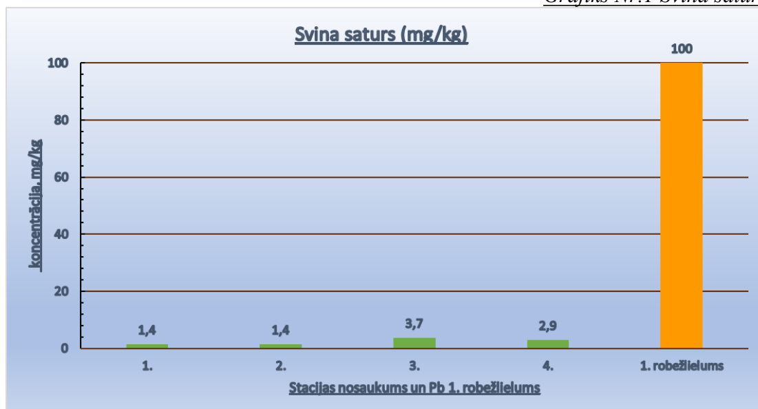
Grafiks Nr.1 Svina saturs
