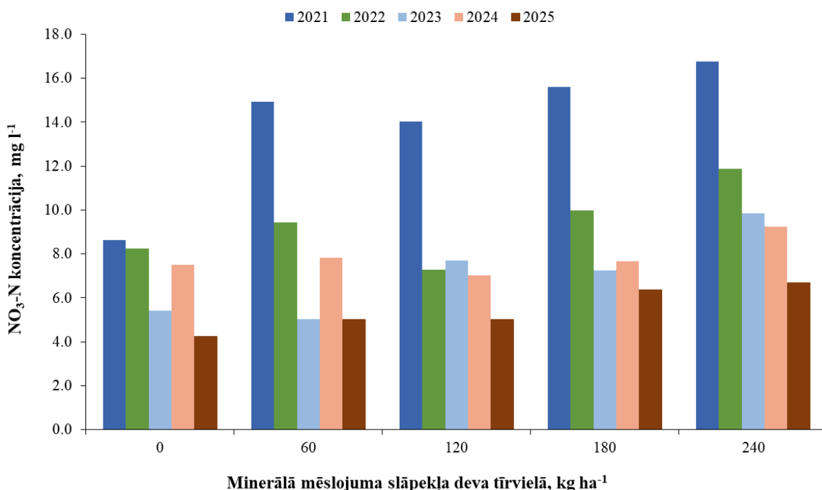
5. attēls. Gada vidējās nitrātu slāpekļa koncentrācijas Mellupītes eksperimentālajos lauciņos (2021.g. – 2025.g.).
