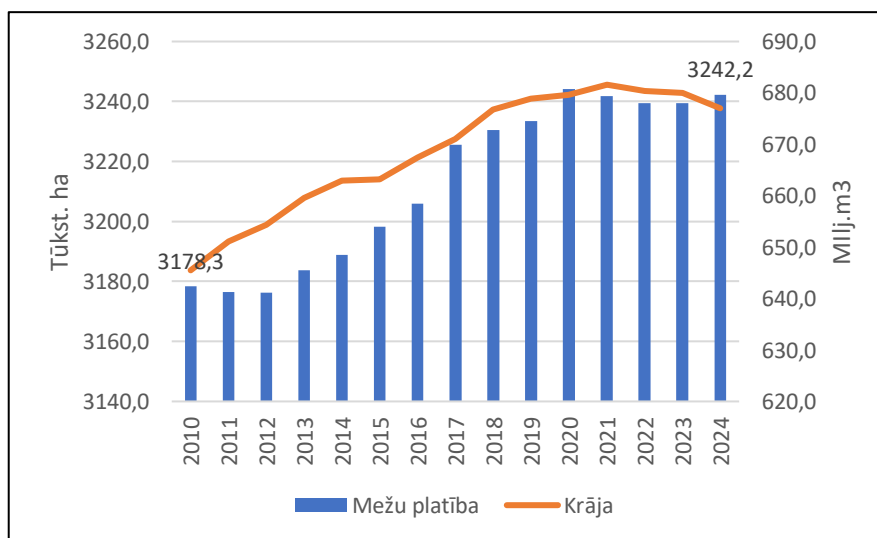
2.2. attēls. Mežu platības un kopkrājas dinamika, 2010.-2024. gads
