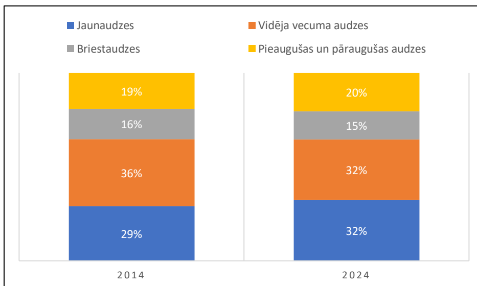
2.4. attēls. Mežu vecuma struktūras pārmaiņas, 2014.-2024. gads
